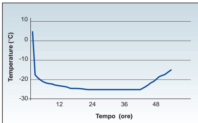
Trasporto di prodotti surgelati (-18°C)
